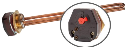
RESISTENCIA + TERMOSTATO GAS-COC-0064 1500 W -CONEXION AL TANQUE 1 1/4" BSPT (41.13 mm) -LARGO DE LA RESISTENCIA: 30 CM APROX -BULBO DE SENSADO EN COBRE -CONTACTOS NA 20 AMP 220 VCA -TERMINALES DE CONEXION FAST-ON PALA MACHO -DIMENSIONES 6 x 270 mm
